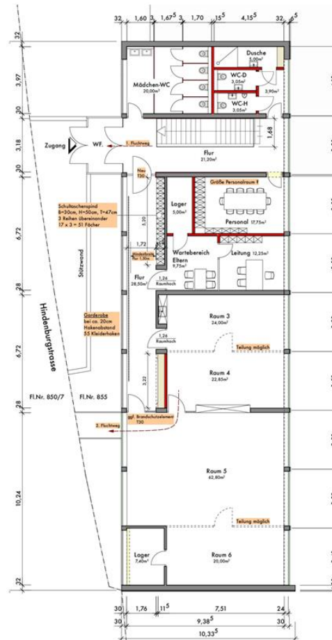
Hort Marktleugast OBERGESCHOSS
