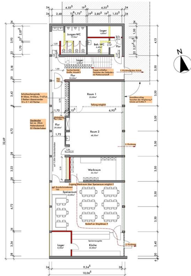
Hort Marktleugast ERDGESCHOSS
